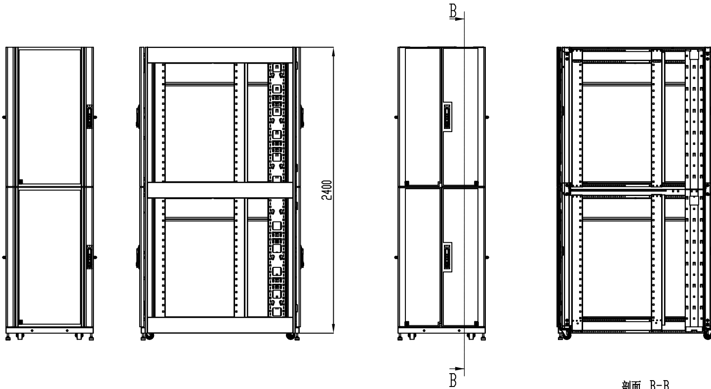
剖面 B-B
